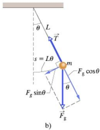
Rys. 16.9. a) Wahadło matematyczne. b) Na ciężarek działają siła ciężkości \vec{F}_g i naprężenie linki \vec{T} . Składowa styczna siły ciężkości F_g \sin \theta powoduje powrót wahadła do położenia równowagi
