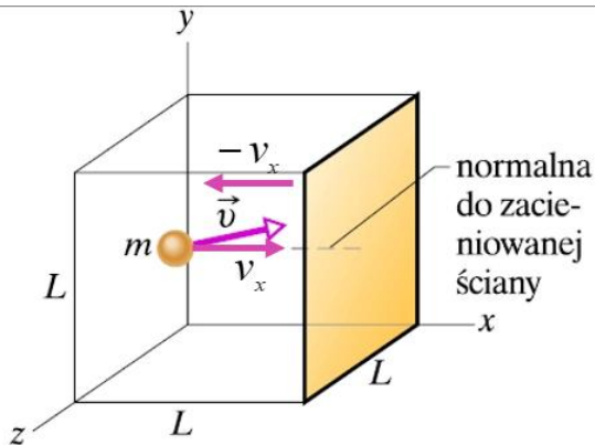
Rys. 20.3. Zbiornik w kształcie sześcianu o krawędzi L zawiera n moli gazu doskonałego. Cząsteczka o masie m i prędkości \vec{v} za chwilę zderzy się z zacieniowaną ścianą o powierzchni L^2 .
