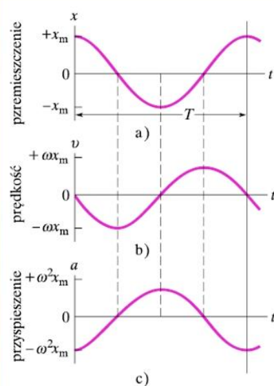
Rys. 16.4. a) Przemieszczenie x(t) ciała wykonującego drgania harmoniczne z fazą początkową \phi równą zero. Jeden pełny cykl drgań wykonywany jest w ciągu okresu T . b) Prędkość ciała v(t) . c) Przyspieszenie ciała a(t)
